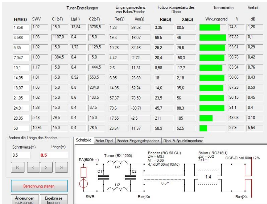
Simulation-Beispiel 160m Windom-Antenne & Sym Tuner HB9BXE
